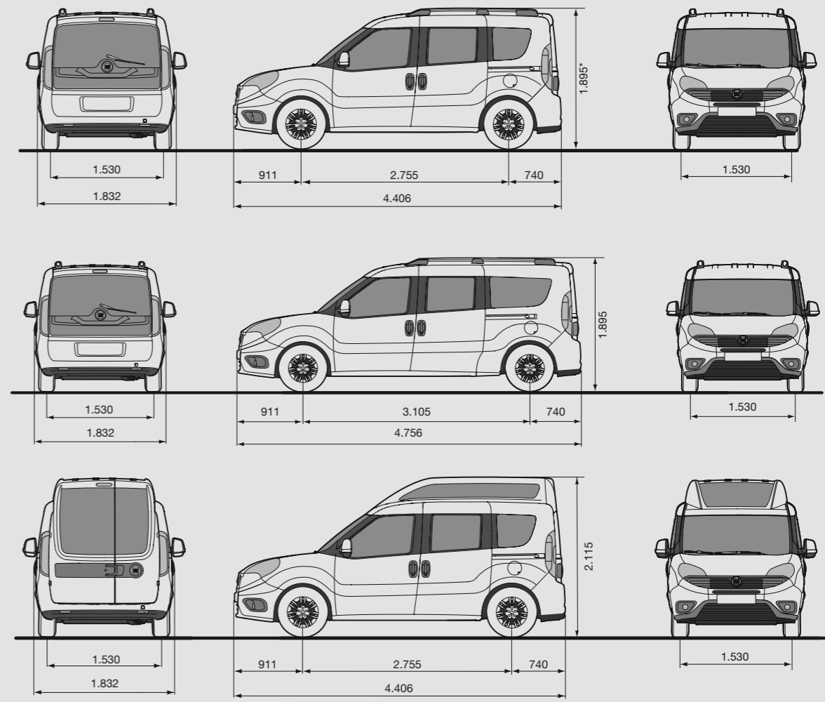
○ = erhältlich - = nicht erhältlich Maßangaben in mm *Trekking +10 mm
